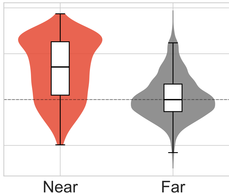
Old slices (***)
